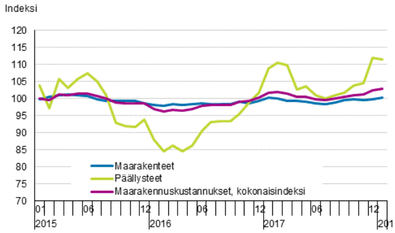
Liitekuvio 1. Maarakennusindeksin 2015=100 kokonaisindeksin, maarakennetöiden ja päällysteiden kustannuskehitys 1/2015–1/2018
